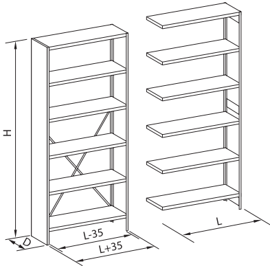
Kuvassa perusosa ja jatko-osa mittoineen.
